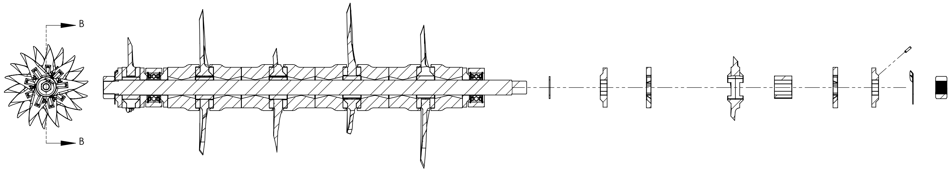
SECTION B-B SCALE 1 : 8
